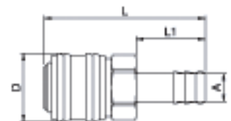
Schlauchtülle
