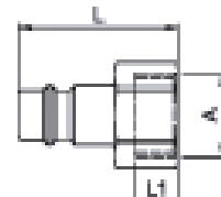
Nippel Innengewinde
