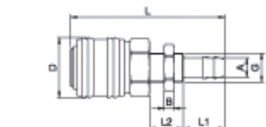
Schottgewinde und Schlauchtülle
