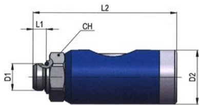
Außengewinde
