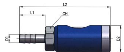
Schlauchanschluss
